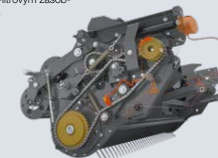
▼ Trvalé mazanie reťazí zberača so 7,2-litrovým zásobníkom oleja.
