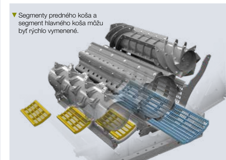
▲ Vymeniteľný segment koša EVION 400.
